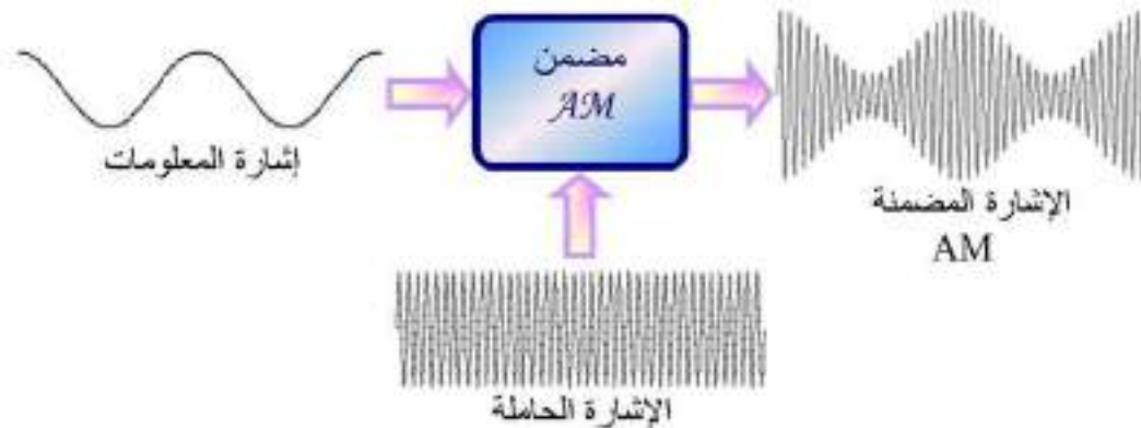
الشكل (4-2) مضمن AM والأشكال الموجية له
