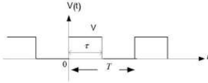
الشكل (1-3) سلسلة النبضات الدورية الغير مضمدة
